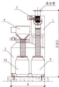
侧面图
