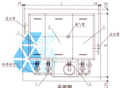
平面图
