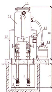
2-2剖面
