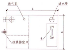
平面图
