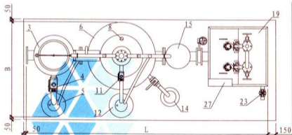
平面图
